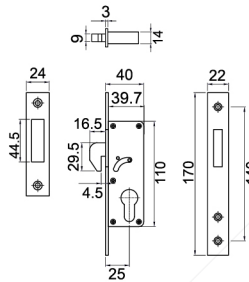
MTS RL DL840 AL F/AL PROFILE SSS
