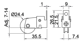
RSW KECIL Capacity (Max) : 25 kg / pairs
