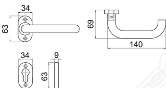
LHTR 84030 OVAL SSS Available : • GUN METAL • MATT BLACK • BLACK PEARL
