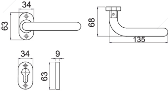
LHTR 0017 OVAL SSS Available : MATT BLACK
