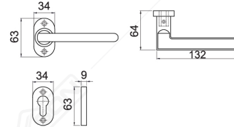
LHTR 0039 OVAL SSS Available : • GUN METAL • MATT BLACK • BLACK PEARL
