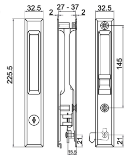
KS J5K ONE SIDE KEY BK Available : • NA • WH • BA
