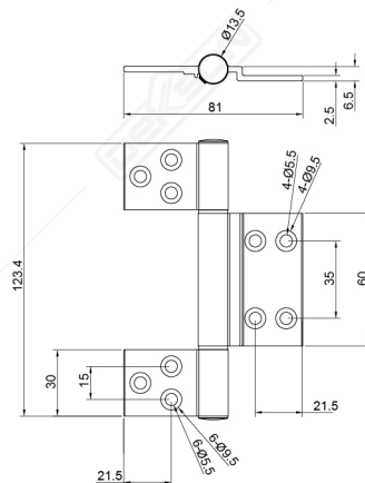
ES AL 8490 BK Capacity (max) : 30 kg / pair
