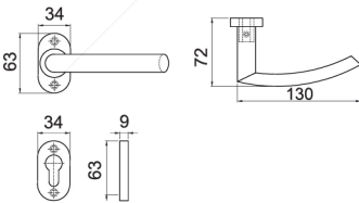
LHTR 0820 OVAL SSS Available : MATT BLACK
